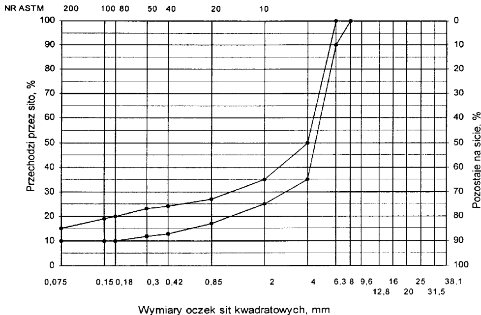
Rys. 1. Krzywe graniczne uziarnienia mieszanki mineralnej SMA od 0 do 6,3 mm do warstwy ścieralnej.
