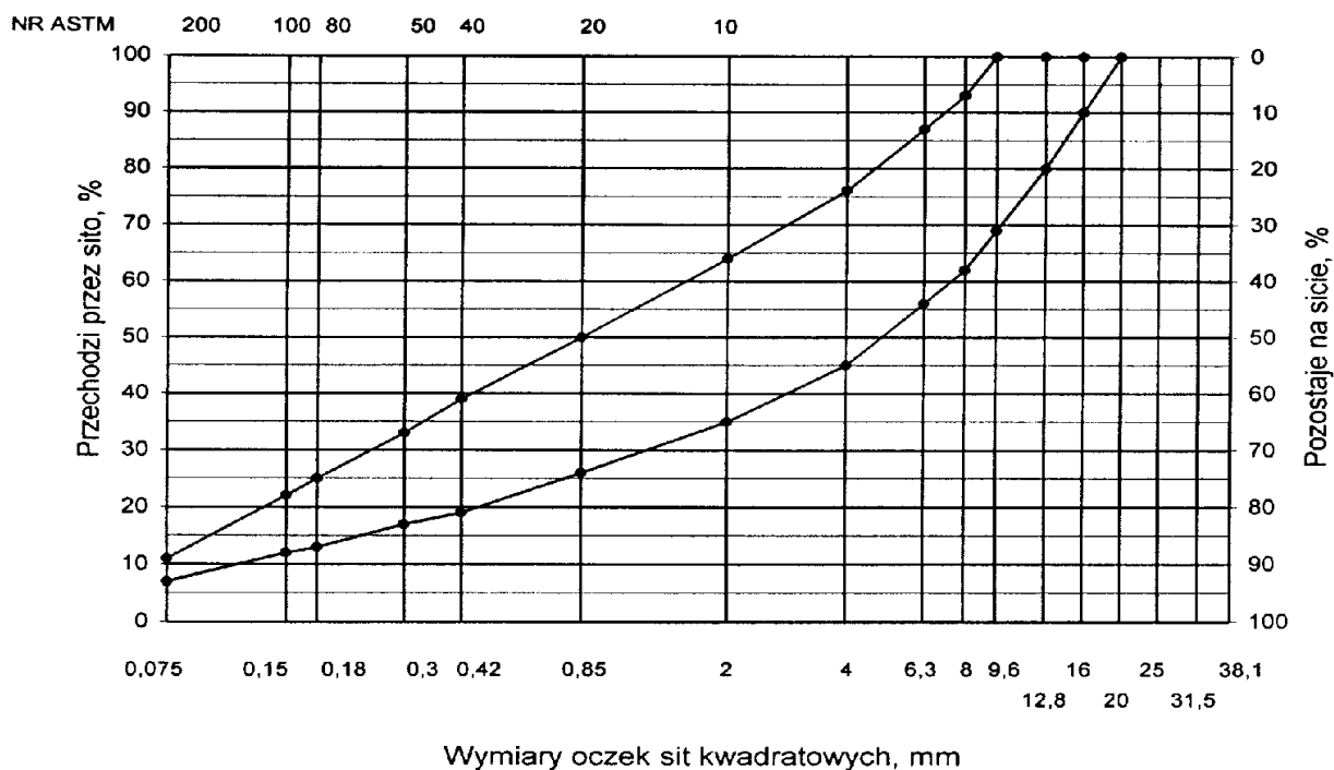
Rys. 1. Krzywe graniczne uziarnienia mieszanki mineralnej BA od 0 do 12,8 mm do warstwy ścieralnej nawierzchni drogi o obciążeniu ruchem KR1.
