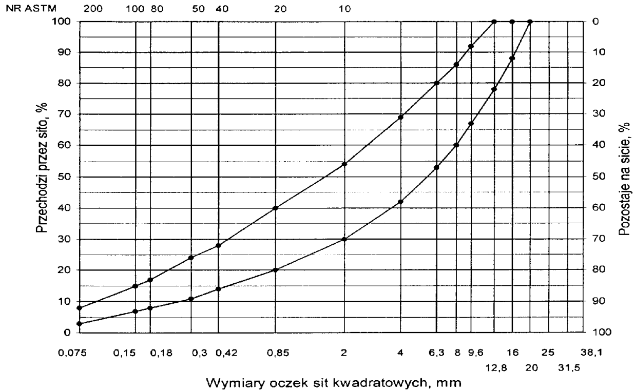
Rys. 2. Krzywe graniczne uziarnienia mieszanki mineralnej BA od 0 do 16 mm do warstwy wiążącej nawierzchni drogi o obciążeniu ruchem KR1
